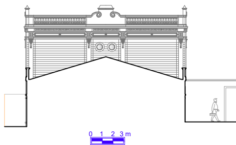
Elevação 02
